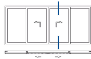
Schema C Detailschnitt vertikal Schiebeflügel, innen
